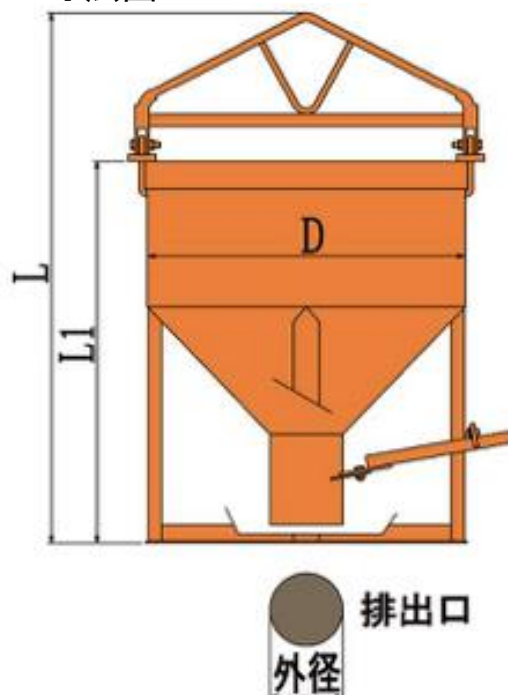
■寸法図
