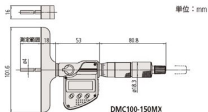
外観寸法図
